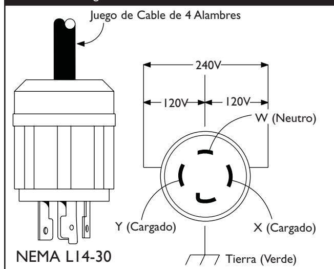
Figura 13 — 120/240 Volt AC, 30 Amp, Receptáculo de Seguridad
